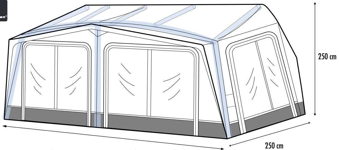
Umlaufmaß/ A-Frame-Size
